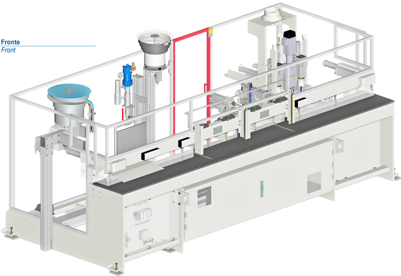
Macchina a CN per foratura, fresatura, pantografatura ed inserimento di colla, spine, ferramenta
